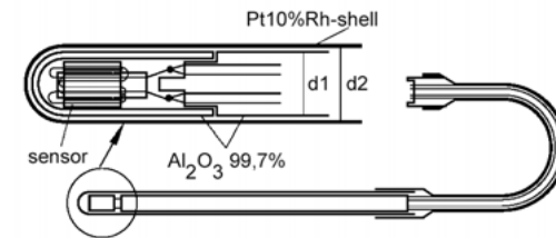
combined thermocouple-noise sensor (source: Physikalisch-Technische Bundesanstalt, Berlin)
